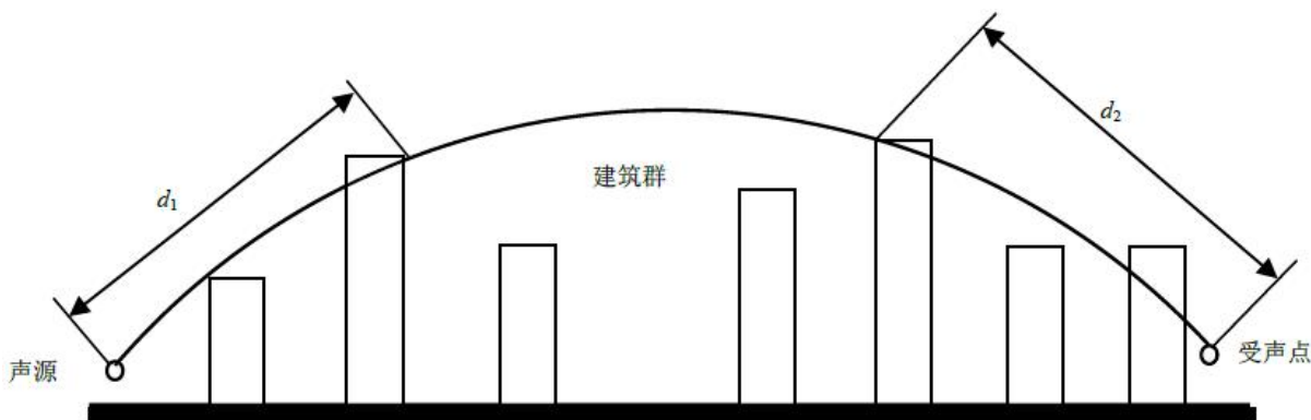
图 4.4-5 建筑群中声传播路径
