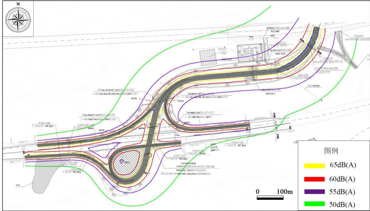
图 4.4-6 互通营运远期昼间等声线图
