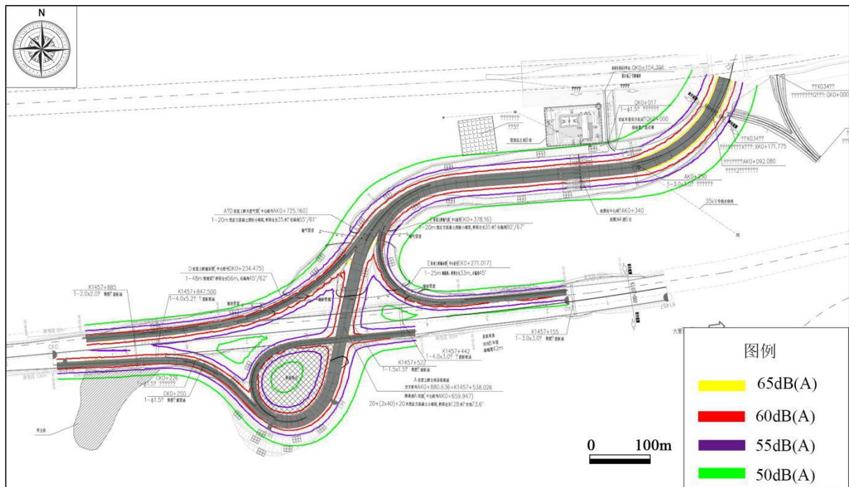
图 4.4-7 互通营运远期夜间等声线图
