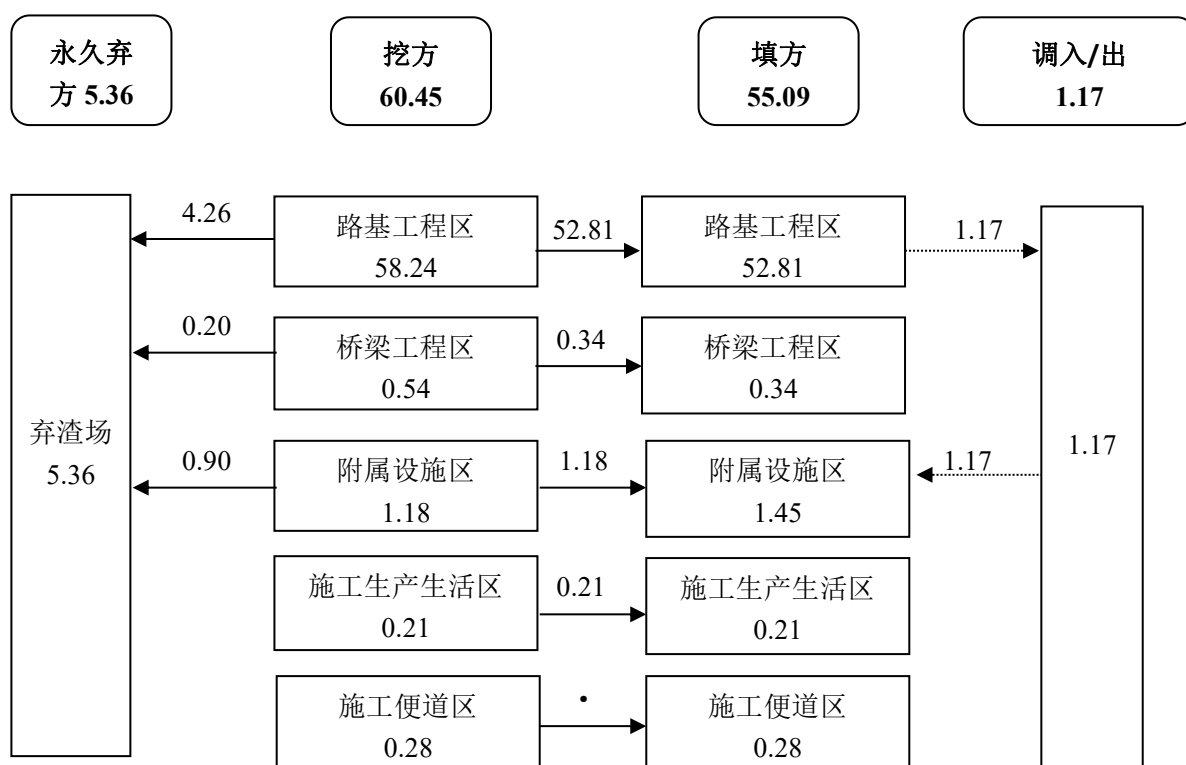
图 2.4-1 工程土石方流向框图 单位：万 m 3
